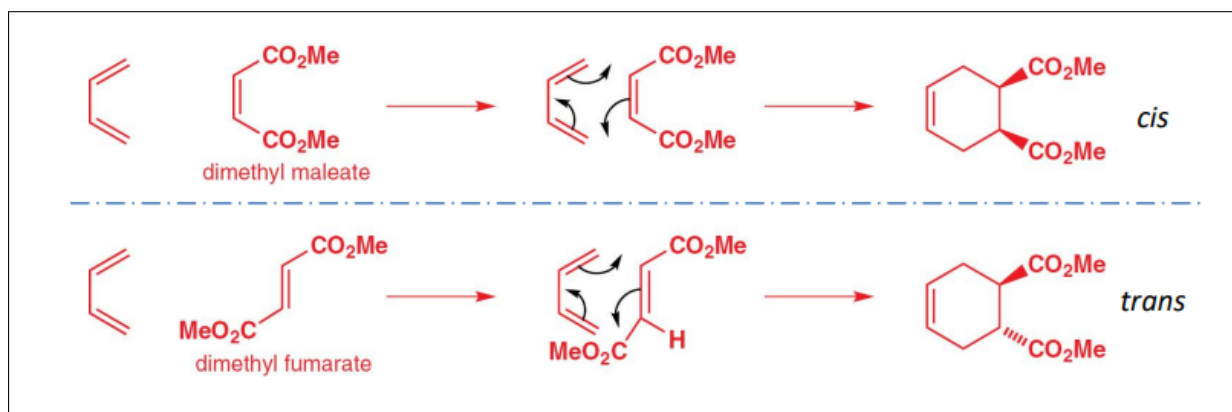
Figura 5: Esempi di reazioni la cui stereochimica è dominata dal dienofilo
