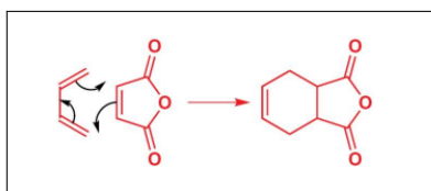
Figura 3: Esempio di reazione di Diels-Alder, notare il movimento a ruota degli elettroni
